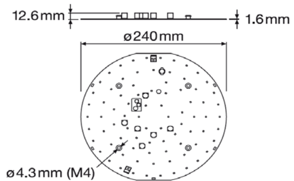
PL-FLAT-AC-SL-G3 2500-840 230V
